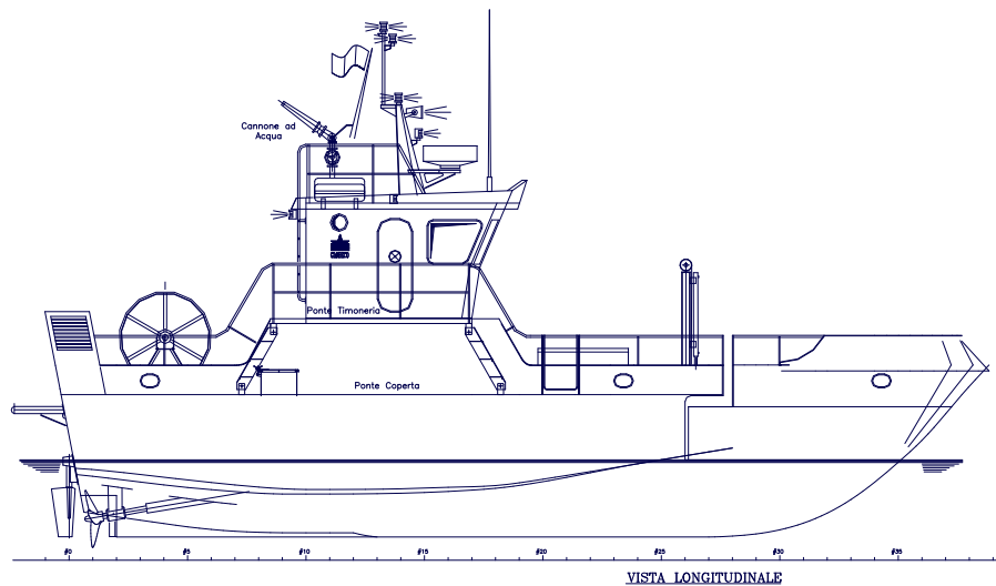
VISTA LONGITUDINALE
