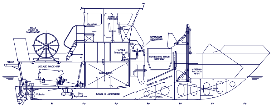
SEZIONE LONG.LE IN MEZZERIA
